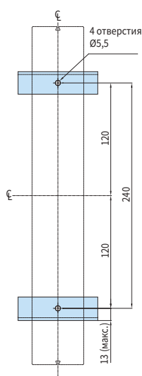
Монтажный чертеж
