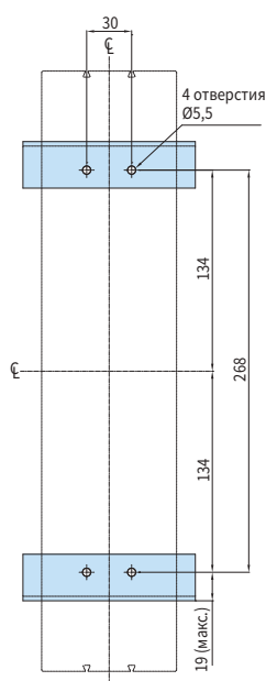
Монтажный чертеж
