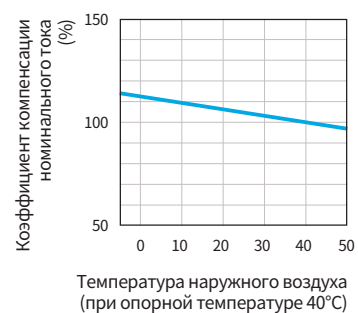
График снижения номиналов по температуре
