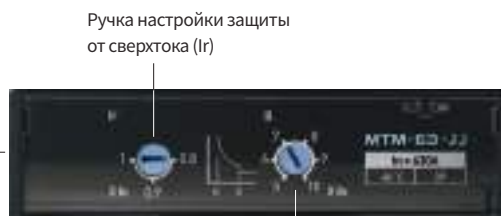
Ручка настройки тока мгновенной защиты ( I_i )
