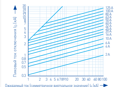
Характеристические кривые тока отключения
