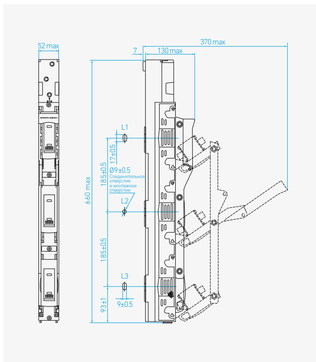
HB-U / 160 AF
