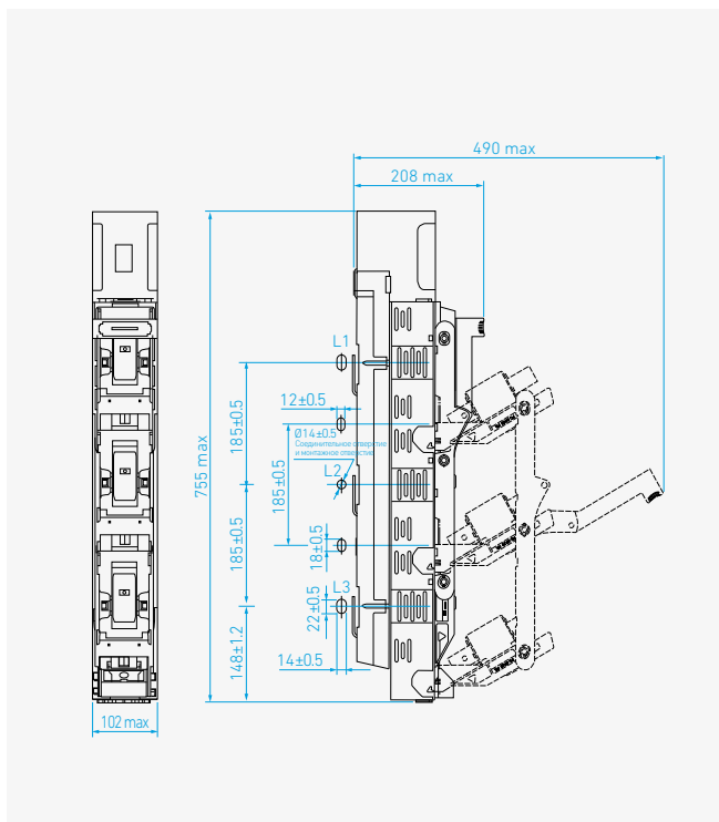
HB-U / 250, 400, 630 AF
